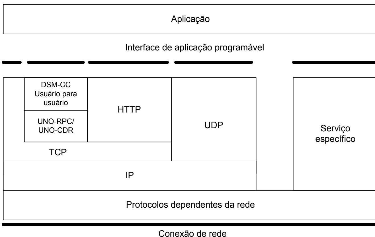
Figura 4 — Pilha de protocolo do canal de interação
