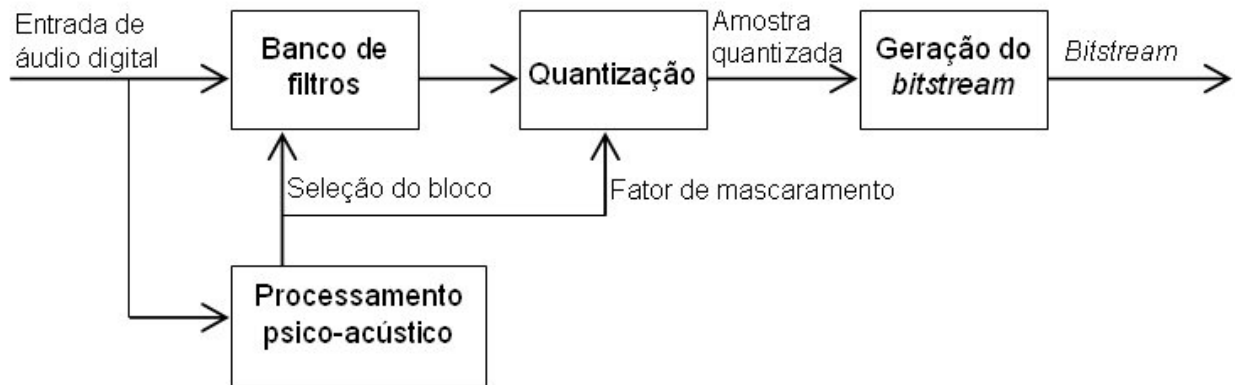
Figura 1 — Procedimentos de transmissão e codificação de áudio
